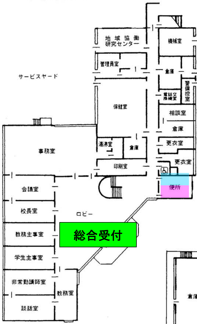
《1階平面図》
