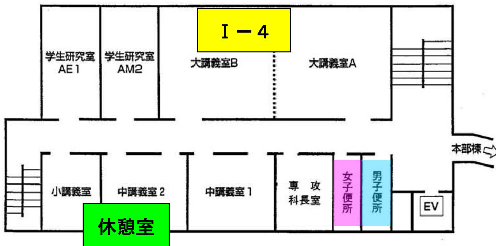
《2階平面図》
