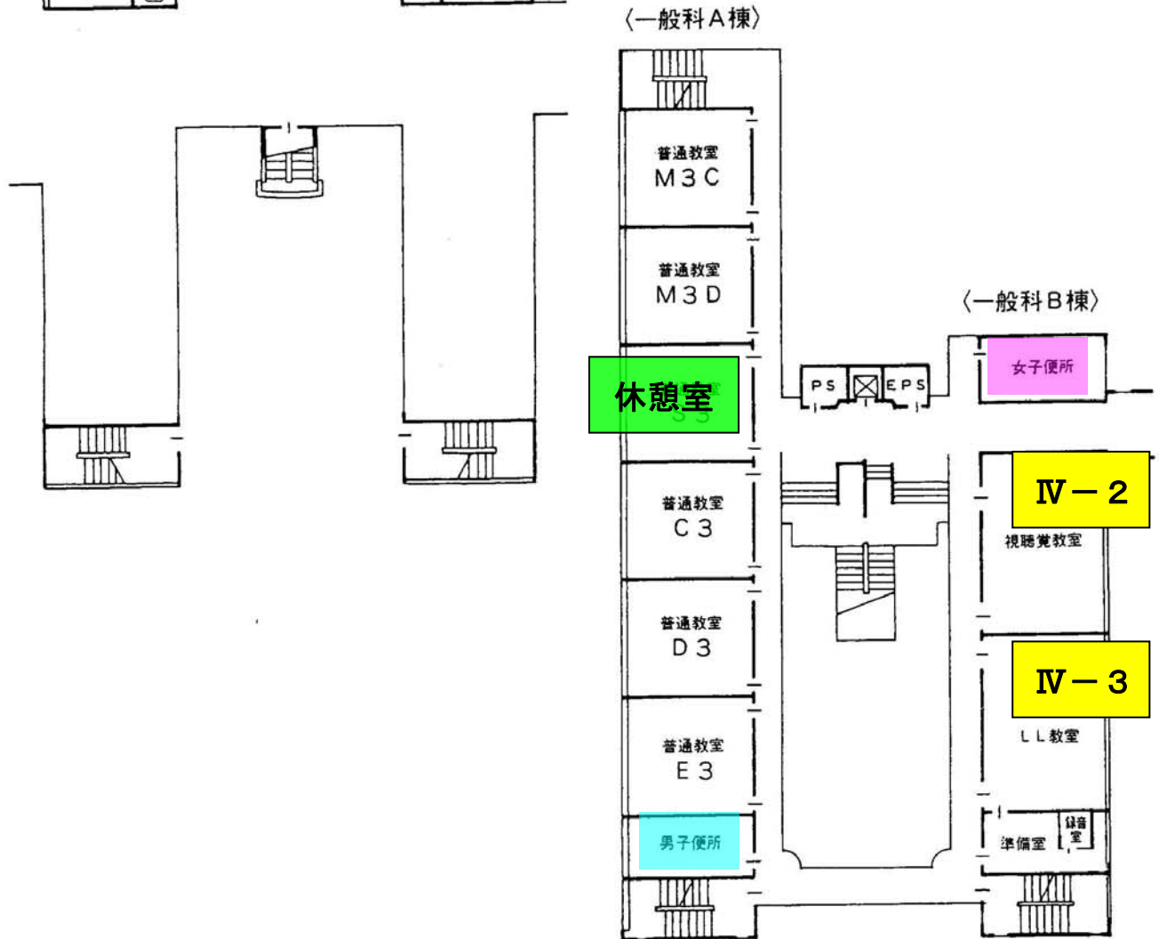
《2階平面図》
